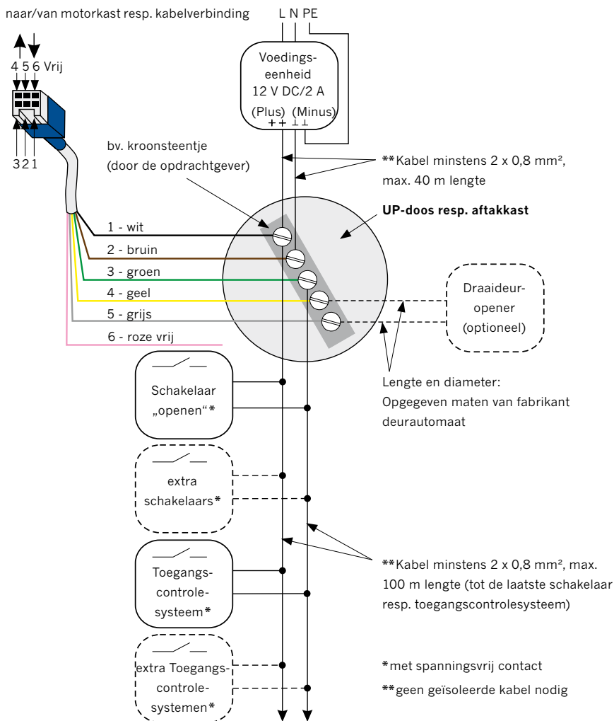
Afbeelding 3.3.1-1: Algemeen aansluitplan
